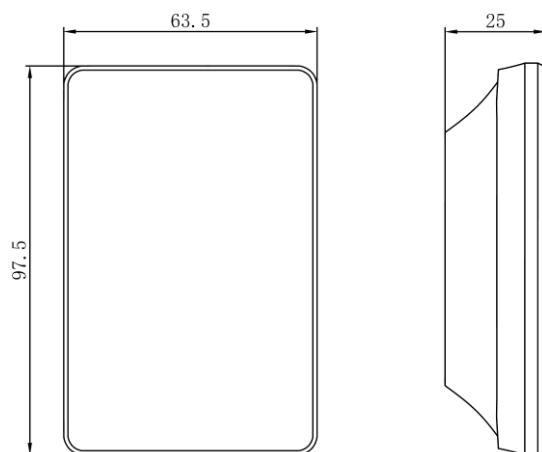
仪表主体外形
