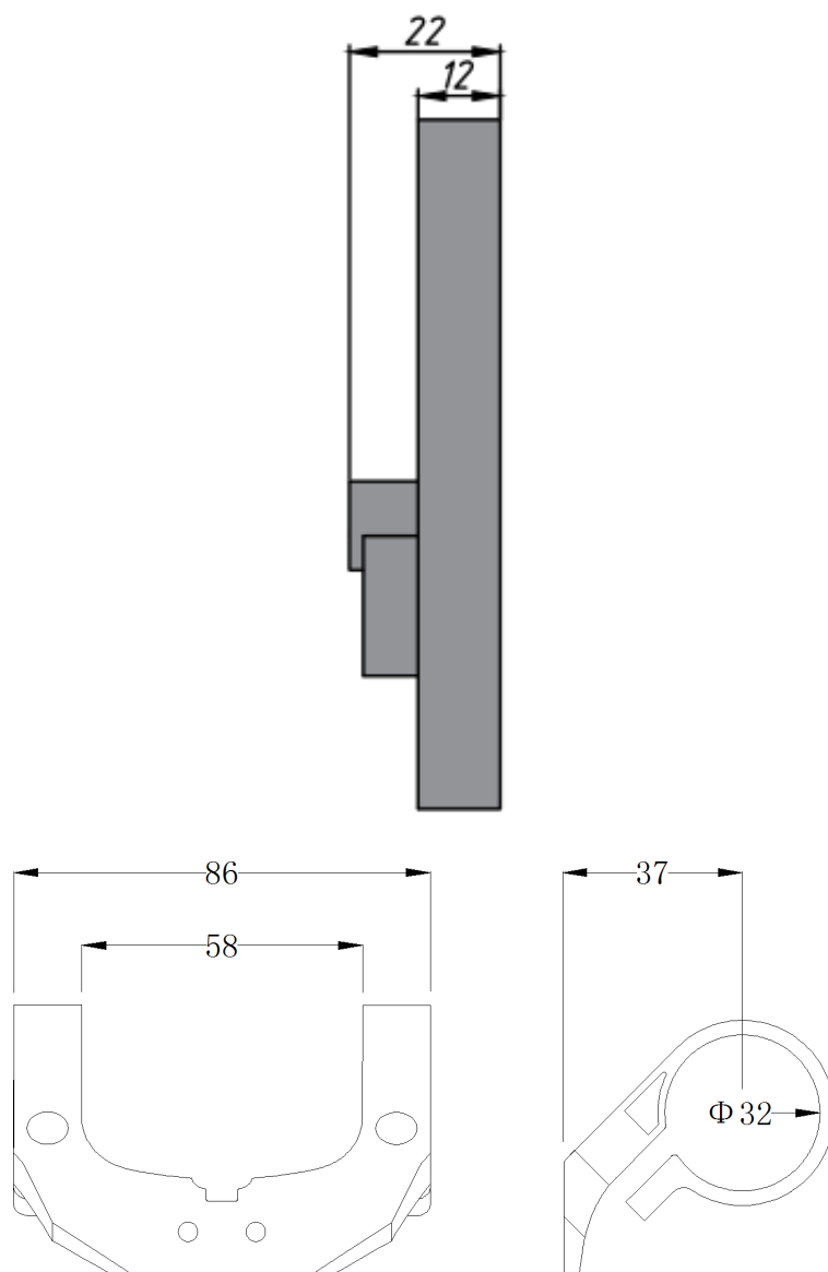
双支架安装尺寸
