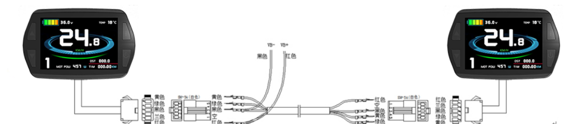
仪表参数复制连线图
