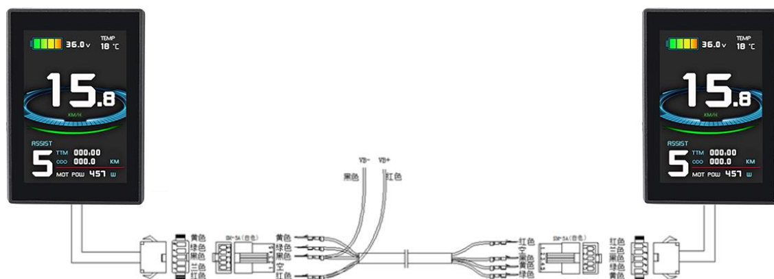
仪表参数复制连线图
