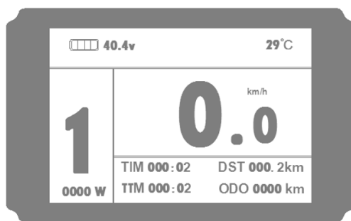
显示界面一
