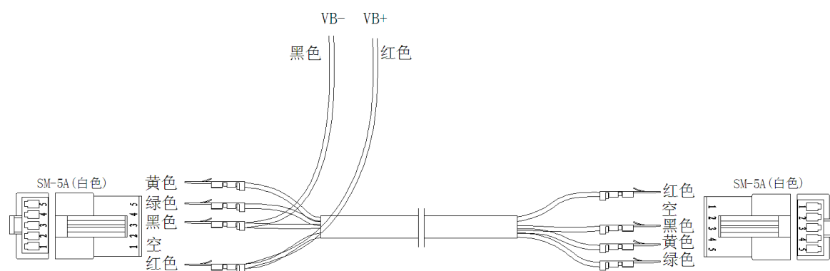
专用连接线
